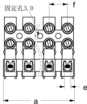
竖插结构
